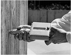
Fig. 2.3 Exécution d'un essai (illustration: modèle NR)
